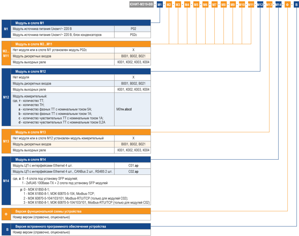
Рисунок А.2 – Код заказа устройства «ЮНИТ-М319-BB»
